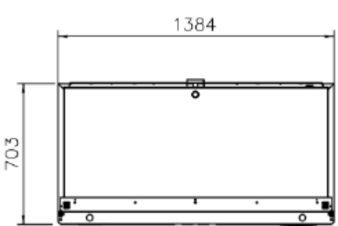
PLANTA/PLAN VIEW/DESSUS/VUE DE PROFIL
