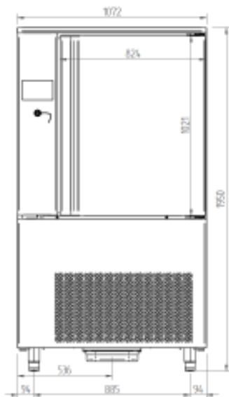
ALZADO/ ELEVATION/ VUE LATÉRAL
