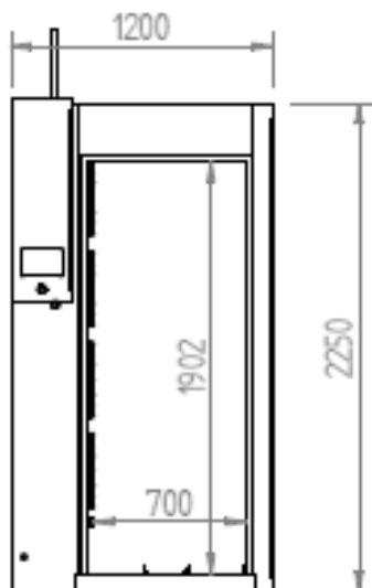
ALZADO/ ELEVATION/ VUE LATÉRAL
