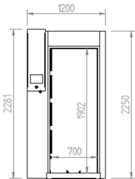
ALZADO/ ELEVATION/ VUE LATÉRAL
