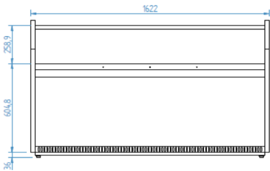
ALZADO/ ELEVATION/ VUE LATÉRAL
