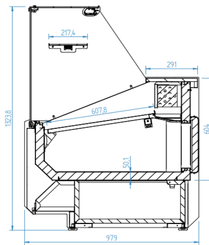
PLANTA/PLAN VIEW/DESSUS/VUE DE PROFIL
